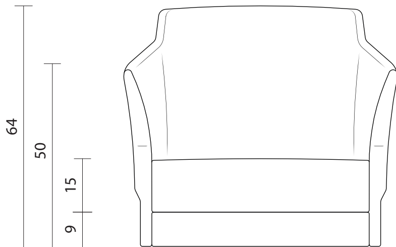
DAKOTA - Scocca poltrona con basamento (PL-DKT-000) (FB-DKT-100) + (SB-DKT-NE)
